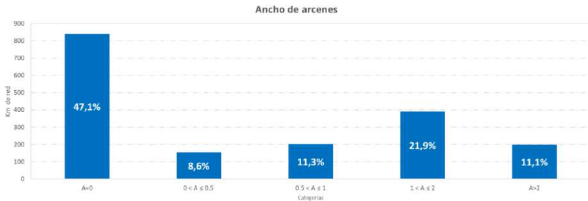
Fig. 61. Distribución de los kilómetros de carretera por ancho de arcén.
