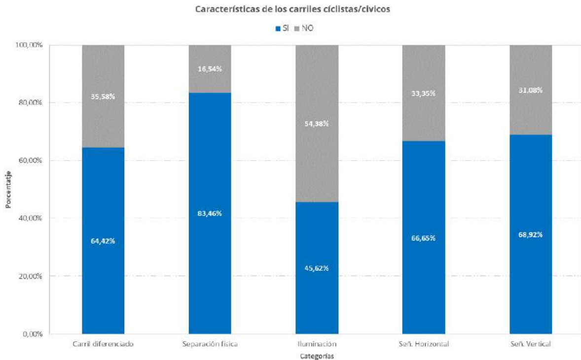
Fig. 65. Porcentaje de elementos identificados en los carriles ciclistas/cívicos (2022).
